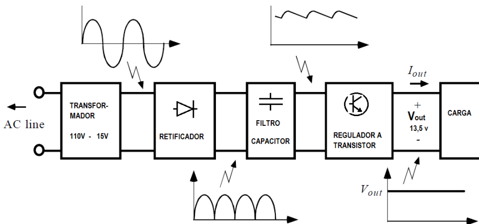
Figura 29 - Diagrama em blocos da fonte de alimentação
