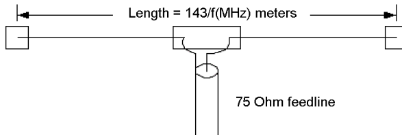
Figura 16 – Diagrama de antena dipolo (figura obtida no Wikipédia)
