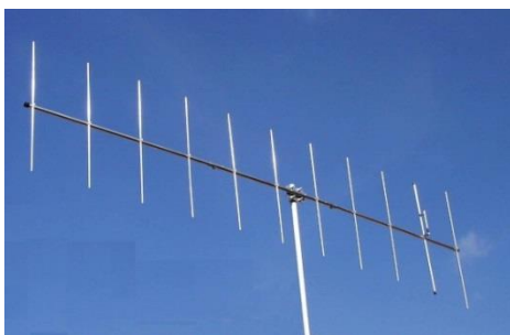
Figura 21 - yagi com 11 elementos para 2m. Como cada dipolo é pequeno (50 cm cada lado) nessa faixa é possível usar antenas com muitos parasitas. Nove diretores e um refletor, porém o direcionamento fica crítico: dez graus cada lado.
