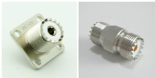
Figura 25 - Conector tipo UHF soquete ou SO-239
