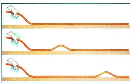
Figura 11 - A ponta livre não faz reflexão. Porém se a ponta estiver fixada numa parede, como na fig. 9, a reflexão será máxima.
