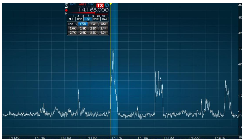
Figura 8 - Exemplo de espectro: podemos identificar doze sinais na tela
