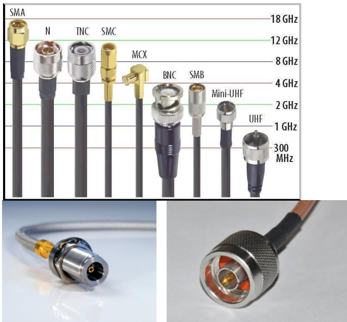
Figura 27 - Conectores tipo "N" nas versões soquete e plug, respectivamente
