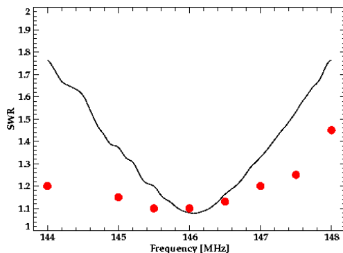
Figura 15 - Gráfico de variação da estacionária numa antena para faixa de 2m. Os pontos vermelhos indicam os valores medidos e a curva marca a estacionária teórica máxima.
