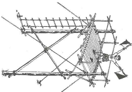
Torre de observação
