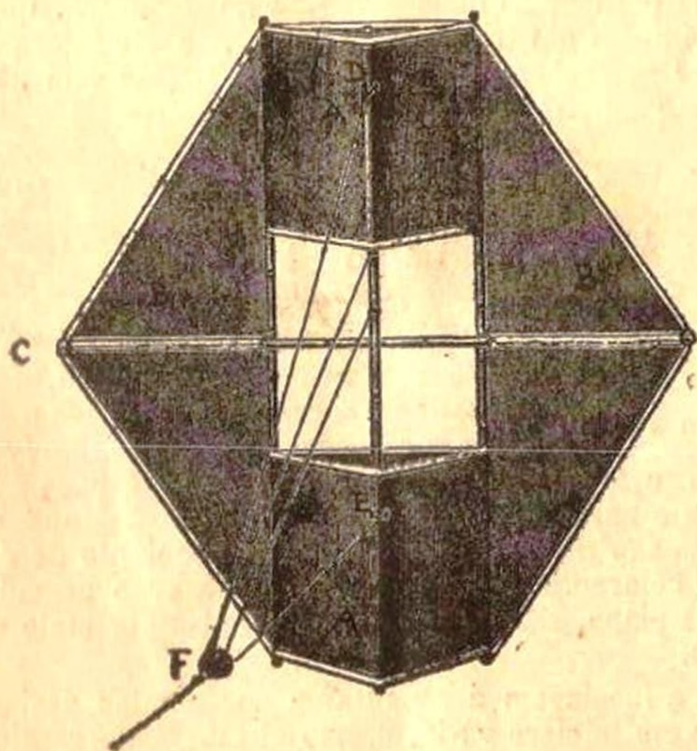
Um papagaio tipo «Conine»
