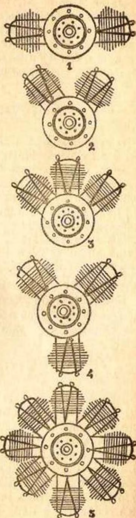
Tipos de motores 1-Horisontal. 2-Em V. 3-Em W ou leque. 4-Em Y 5-Em estrela.
