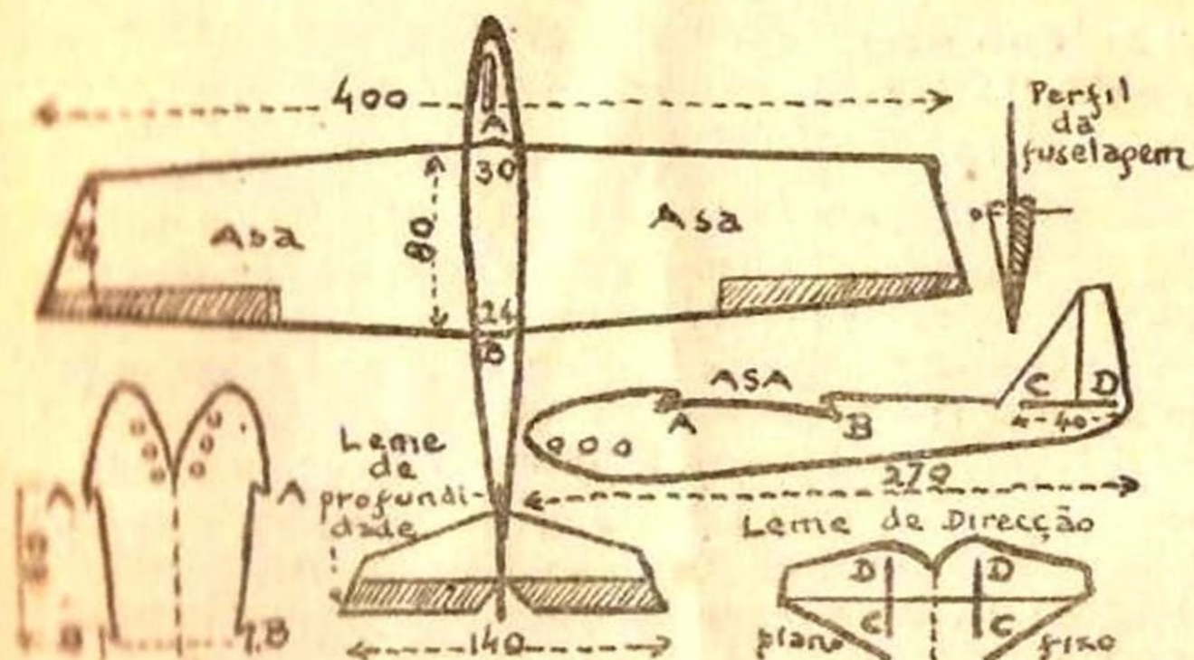
Planta d'um modêlo de «planeur» (Medidas em milímetros)
