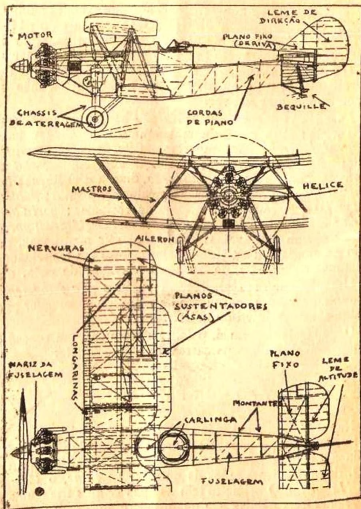
Planta dum avião
